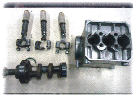
ポンプ内焼付け破損写真
