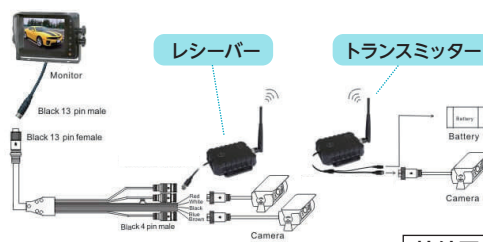
接続図
